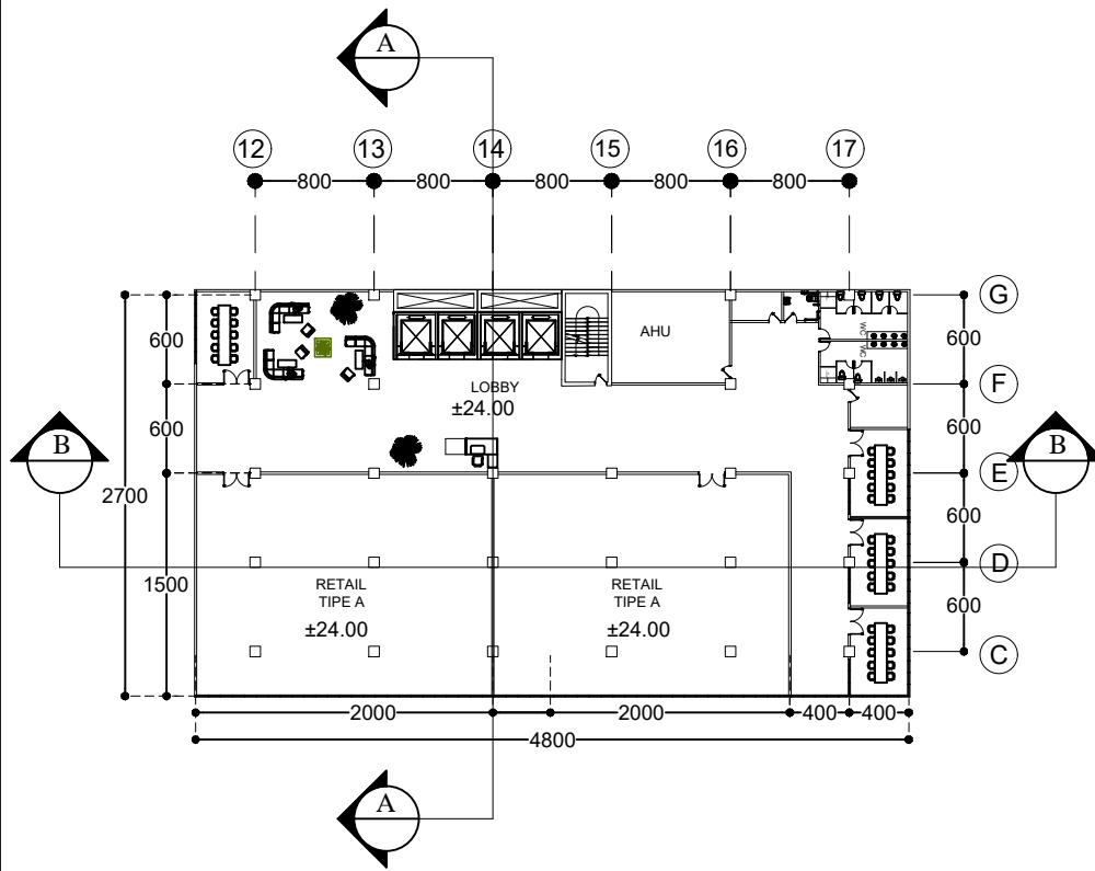
SCALE BAR 1:200 DENAH OFFICE LT 2 dan 3
