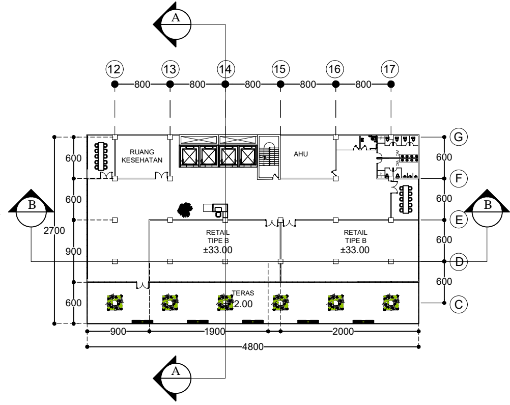
SCALE BAR 1:200 DENAH OFFICE LT 4 dan 5
